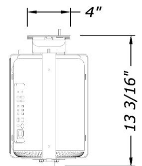
ELEVATION
