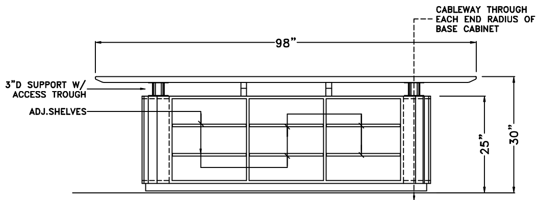
ELEVATION
