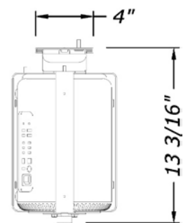
ELEVATION
